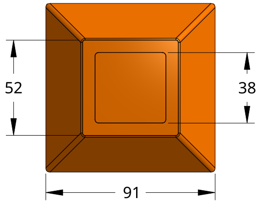
Top SCALE 1:2
