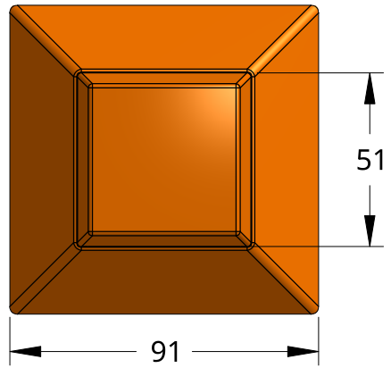
Top SCALE 1:2
