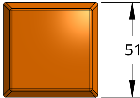
Top SCALE 1:2
