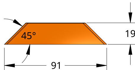
Right SCALE 1:2
